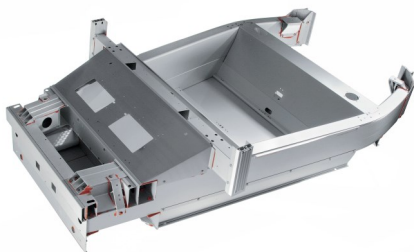
Verlijmde aluminium chassis van de Lotus Elise
