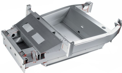
Verlijmde aluminium chassis van de Lotus Elise
