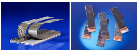
Lijmproofstukken ten behoeve van een peltest (links) en afschuiftest (rechts)
